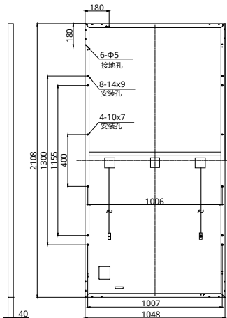
背面图
