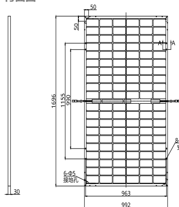
背面图
