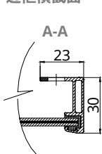
安装孔
